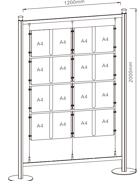
FS-02(1200x2000)A4
