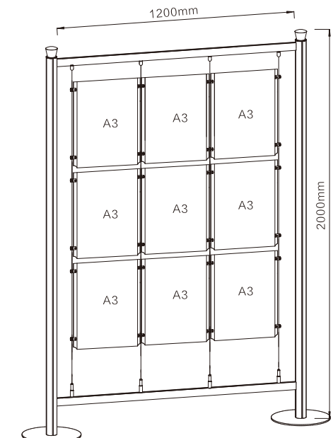
FS-02(1200x2000)A3
