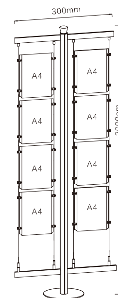
FS-02(300x2000)A4
